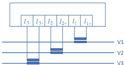
نحوه اتصال جریان سه فاز:
