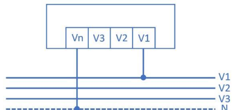
نحوه اتصال ولتاژ تکفاز:
